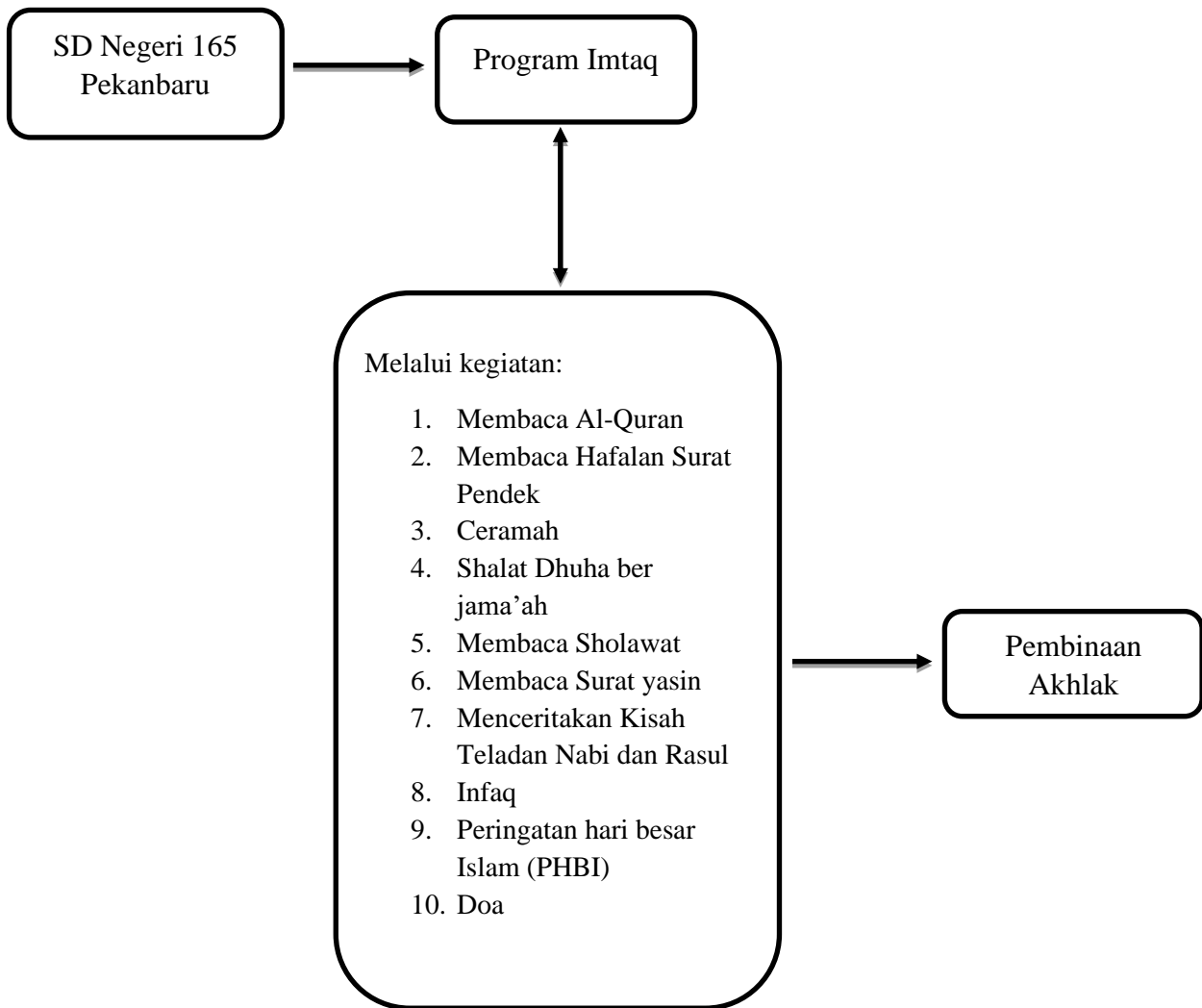
Gambar 2.1 Kerangka Berfikir
